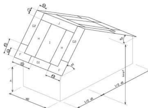
4. Ongelijkzijdig zadeldak
