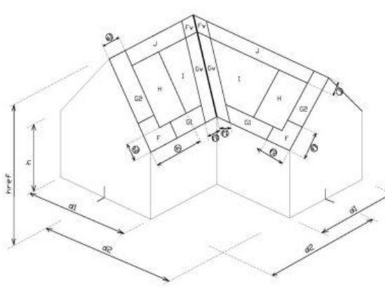
8. Zadeldak met hoek- en kilkeper
