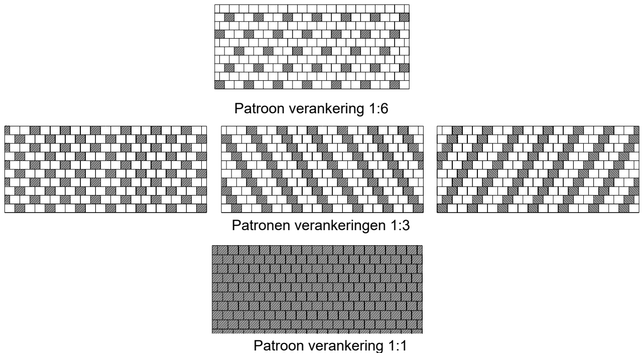
Figuur 1: Verankeringsschema's en patronen
