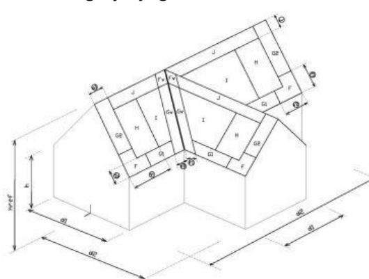
6. Zadeldak met nok haaks doorlopend
